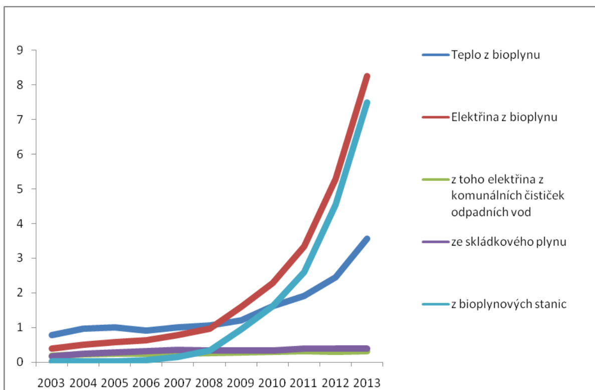
Graf č. 3: Použití bioplynu a původ bioplynové elektřiny v letech 2003 – 2013 podle studie Energická krajina (na levé škále je vyrobená energie v petajoulech ročně)
